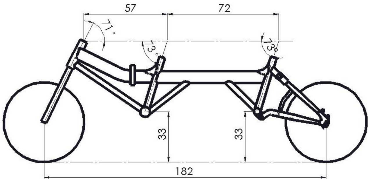
Abbildung 1: Geometrie
